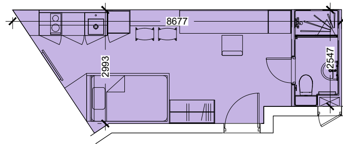
SINGLE BEDROOM Type 02E
